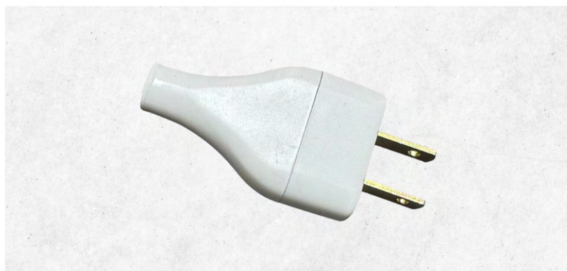
Enchufe c/tapa protectora y espigas planas 16A-250V blanco
